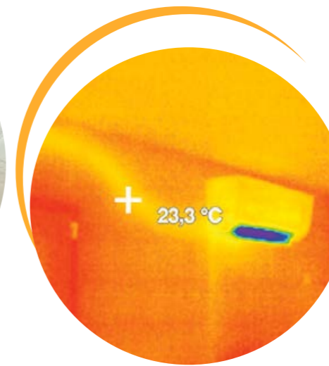
Thermografie Aufnahme einer Klimaanlage mit sichtbaren Unterputz Kältemittelleitungen
